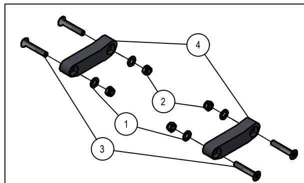
Glijsloten looprol
