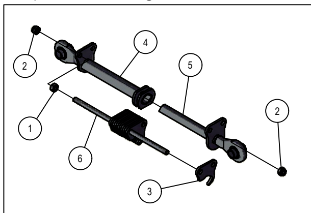
Looprol verstelling
